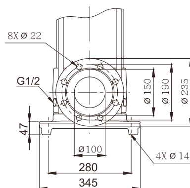
Flange (DIN) PN25-40 / DN100
