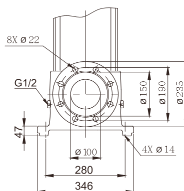
Flange (DIN) PN25-40 / DN100
