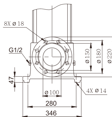
Flange (DIN) PN16 / DN100
