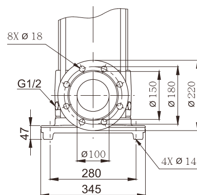
Flange (DIN) PN16 / DN100
